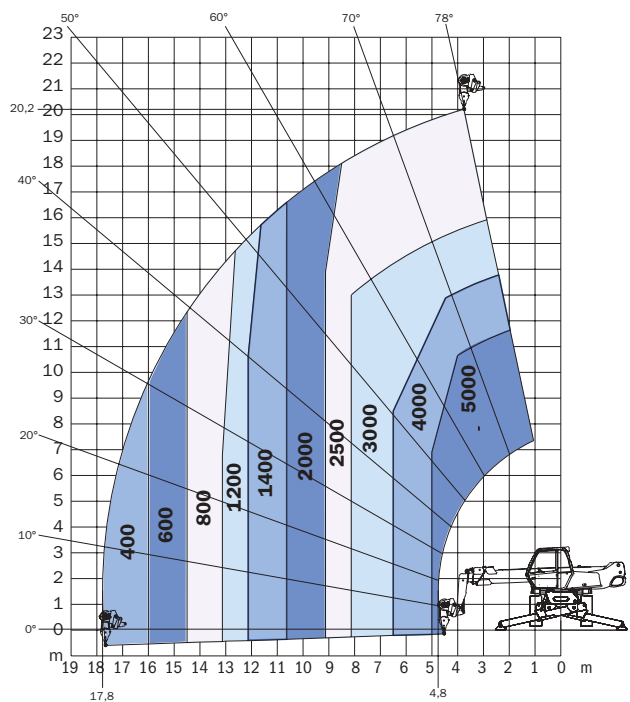
ABGESTÜTZT MIT SEILWINDE 5 T
