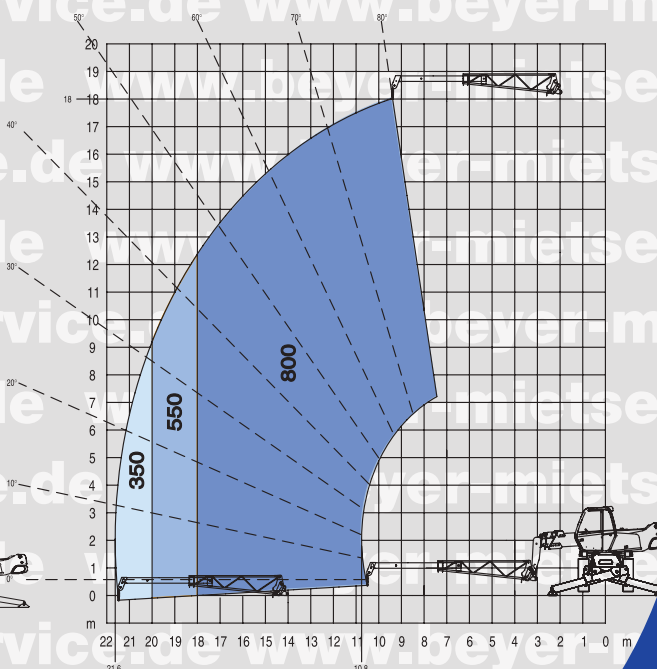
ABGESTÜTZT MIT TELESKOPIERBAREM KRANARM
