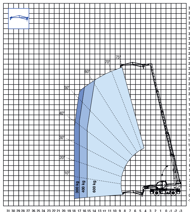
Gittermast 0,6 t / 4,2 m - auf Reifen
