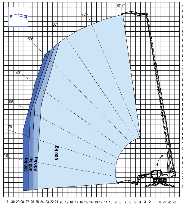
Gittermast 0,6 t / 4,2 m - auf Stützen
