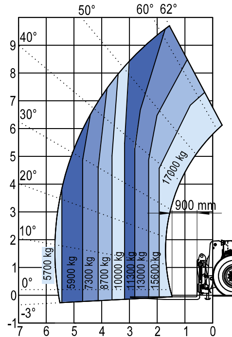
Lastschwerpunkt 900 Millimeter
