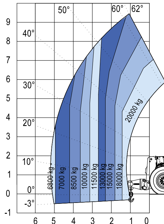
Lasthaken 20 Tonnen
