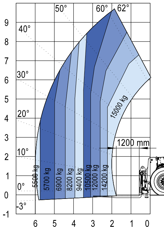
Lastschwerpunkt 1200 Millimeter
