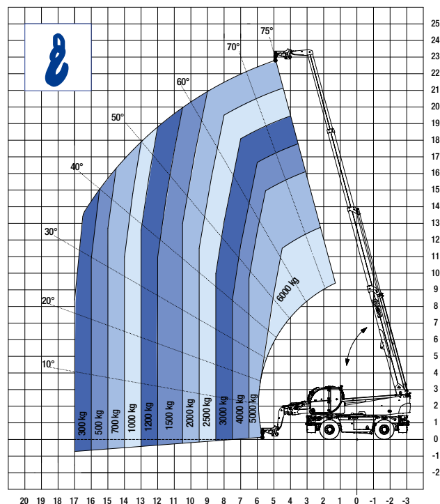
Lasthaken 8 t - auf Reifen
