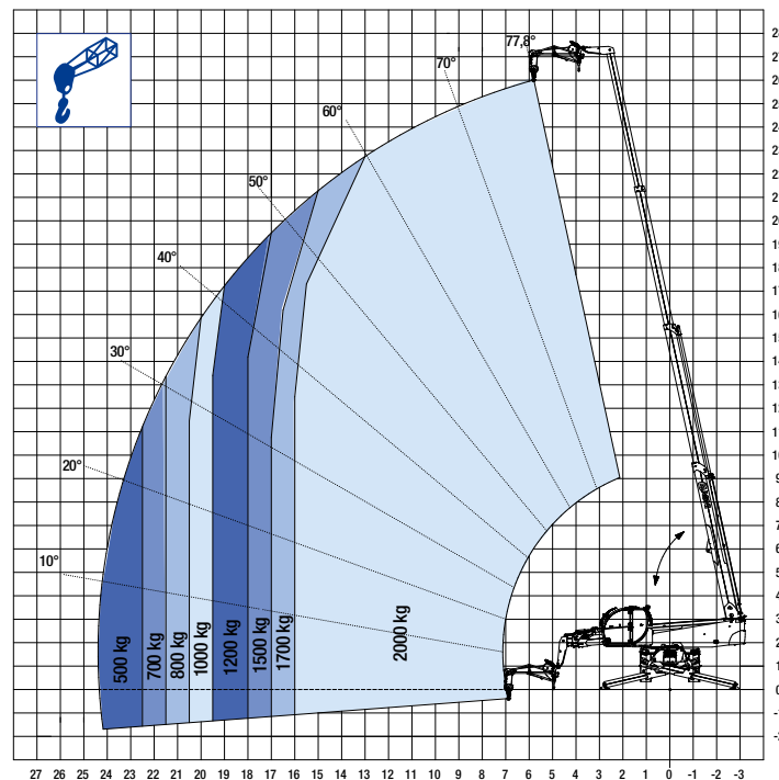
Gittermast mit Winde 2t - auf Stützen
