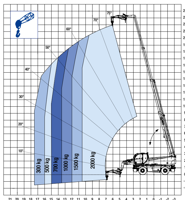
Gittermast mit Winde 2t - auf Reifen
